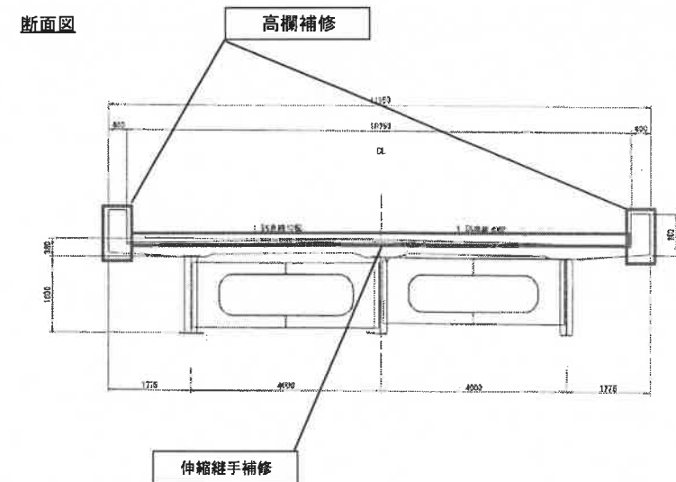
断面図
